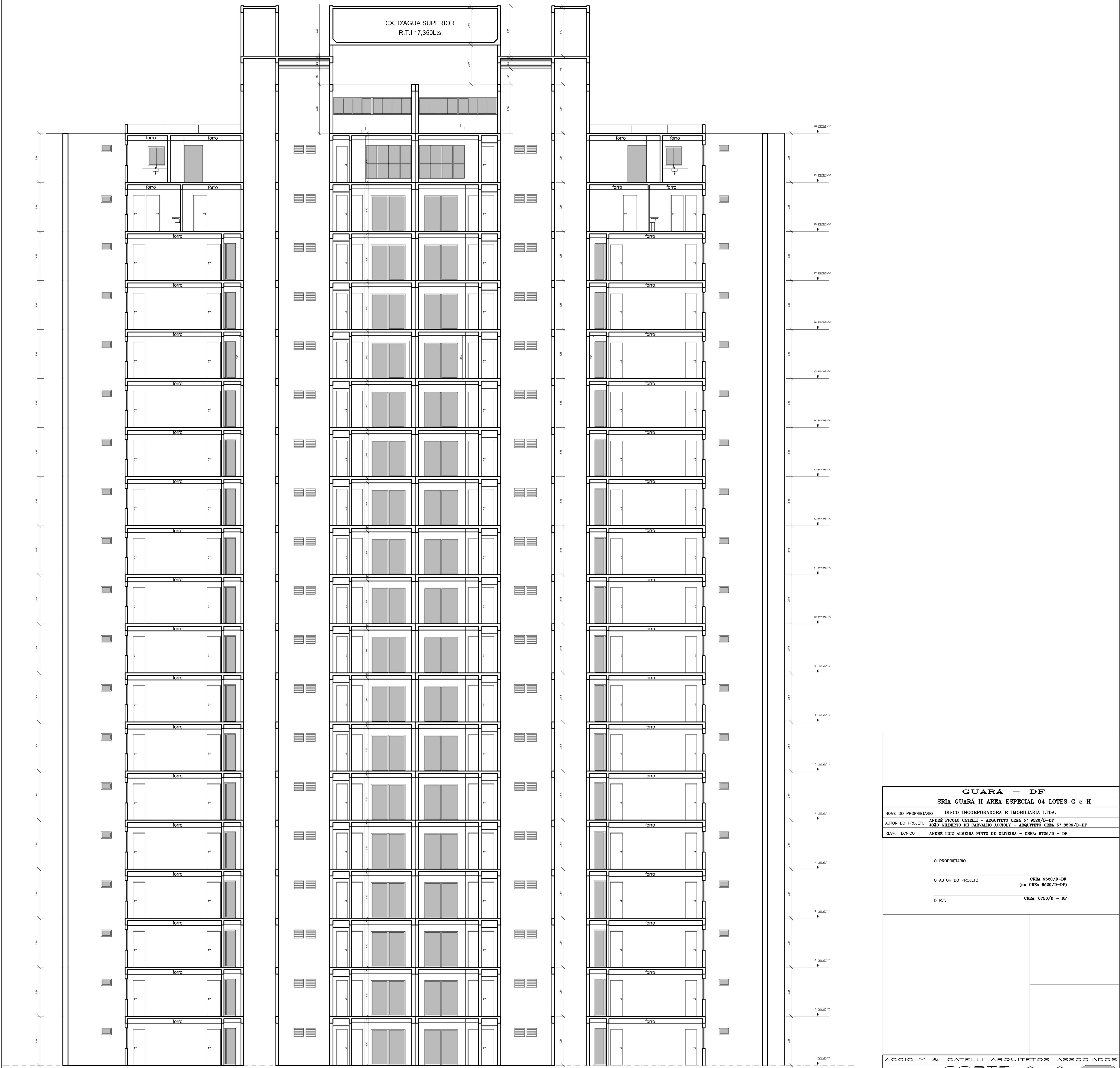
CORTE A-A ESCALA 1:100
